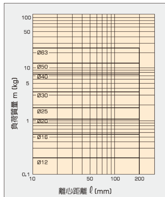
● (D) 50行程以上, V = 400mm/s
