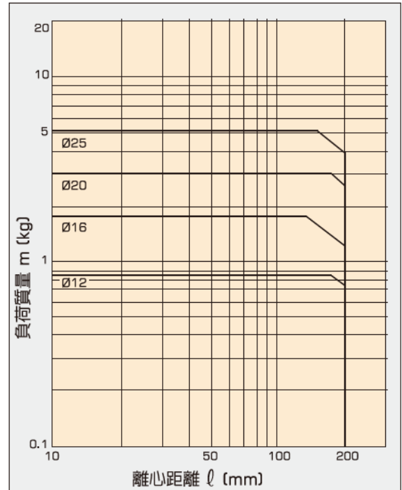
● (F) 30行程以上, V = 200\text{mm/s}
