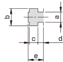
B 部詳圖, 比例 2:1
